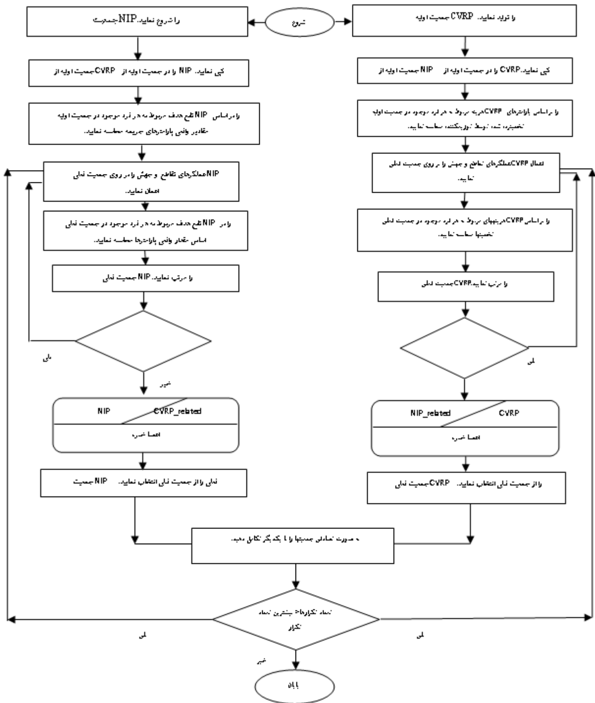
شکل ۵. فلوجارت مربوط به الگوریتم تکامل تدریجی دوسطحی برای NIHVPR با اطلاعات نامتقارن
