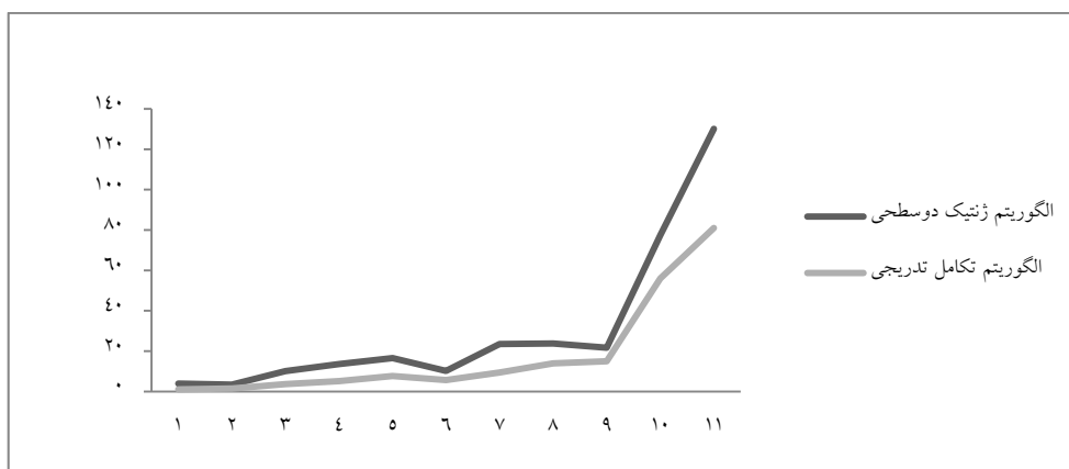
شکل ۸. مقایسه بین دو الگوریتم فراابتکاری توسعه داده شده بر اساس زمان محاسباتی (بر حسب ثانیه)
